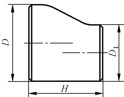
b) 偏心异径管
