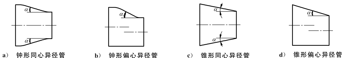
图 B.1 异径管(同心和偏心)斜边与轴线的夹角 \alpha 示意图
