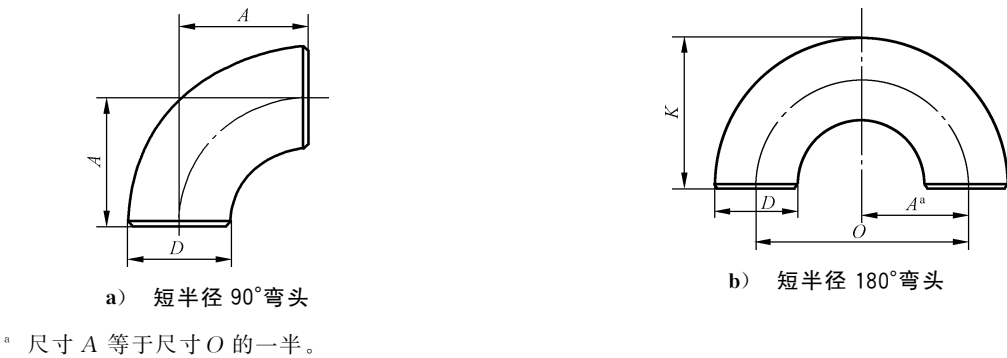
图 3 短半径 90°和 180°弯头形状
