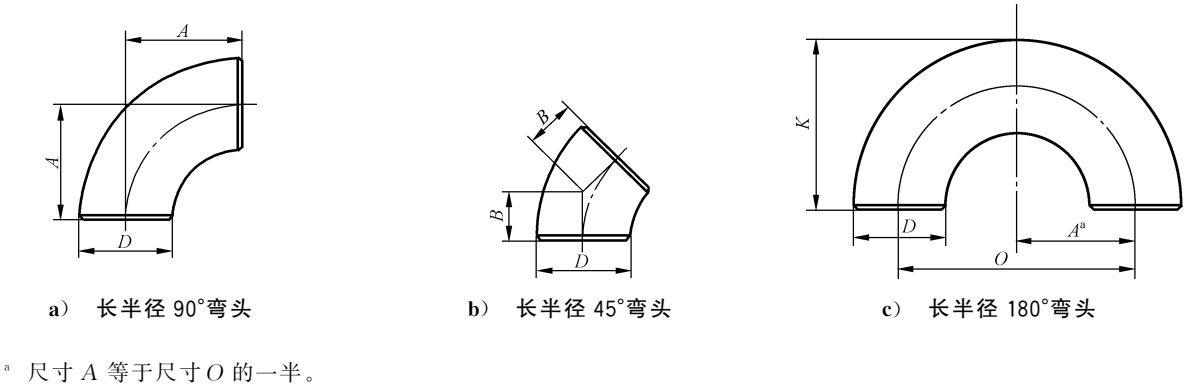
图 1 长半径 90°、45°和 180°弯头形状
