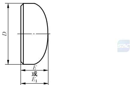
图 8 管帽形状
