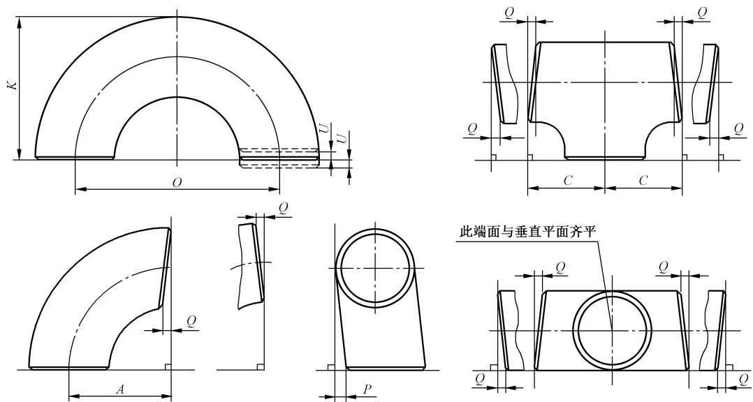
图 12 公差简图
